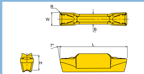
ID Grooving
