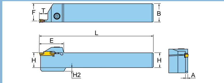
OD Profiling
