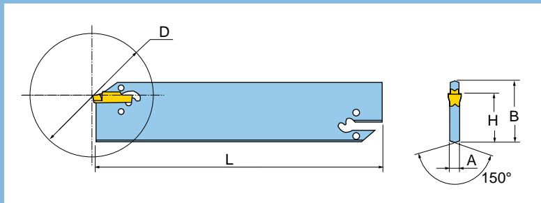
OD Grooving
